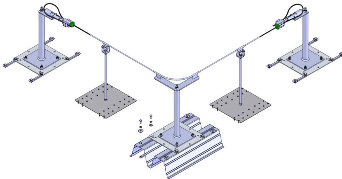
Seilsystem auf Trapezdach
