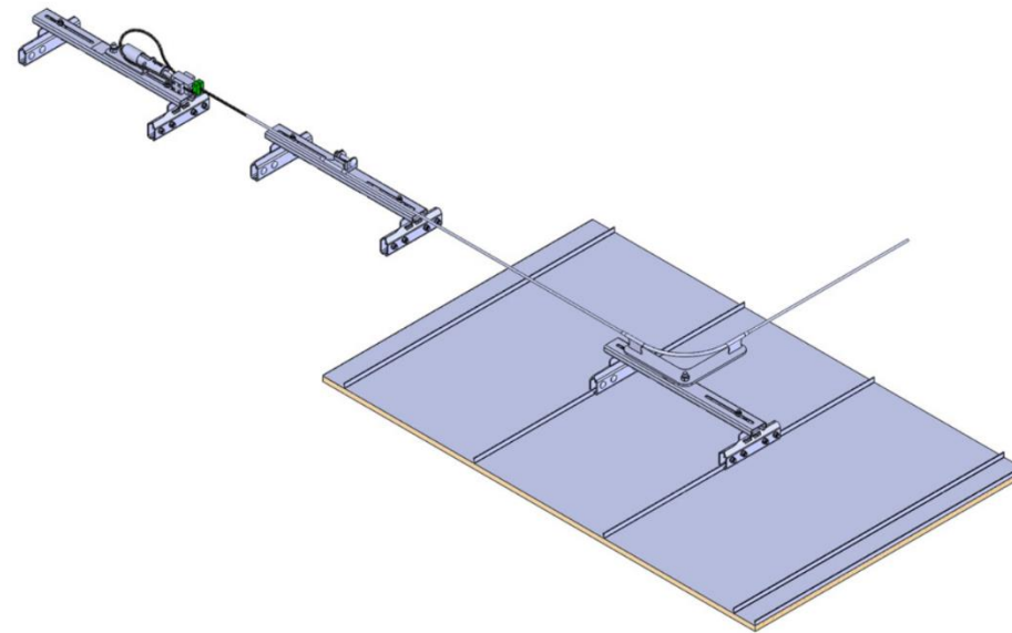
Seilsysteme auf Kalzip- / Stehfalzdach
